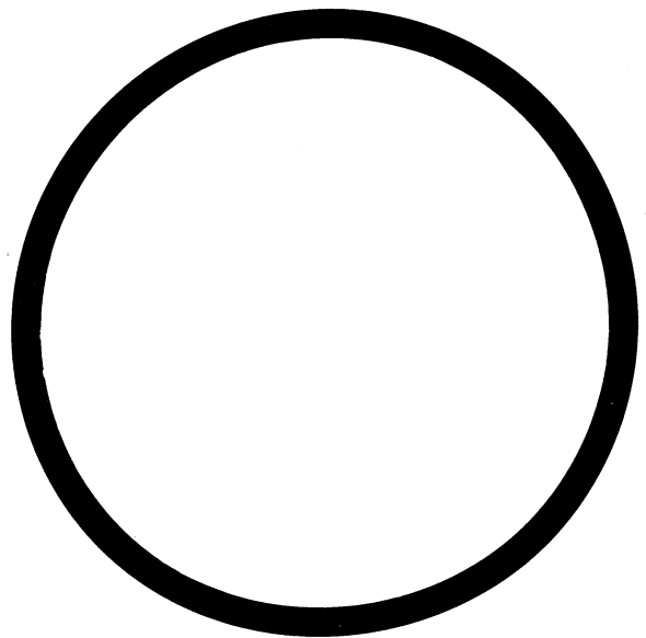
PN 00-3084-59 2.750 I.D. X 3.00 O.D. x 0.134 TETRASEAL/BUNA-N
