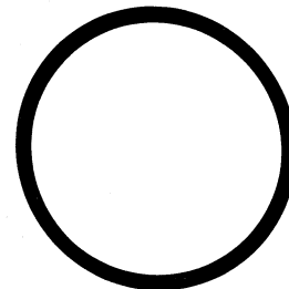
PN 00-3310-76 1.187 I.D. X 1.312 O.D. x 0.062 TETRASEAL/BUNA-N
